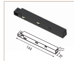
48V-Q1/Q2 END FEED
